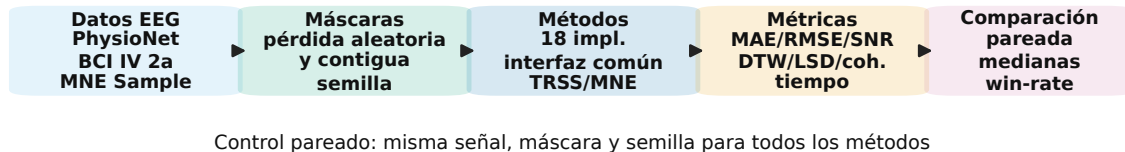
Figura 3.1: Flujo metodológico de evaluación con control pareado. Cada método se aplica sobre los mismos conjuntos de datos, máscaras de pérdida y semillas; luego se calculan métricas de reconstrucción y costo antes de comparar los métodos por escenario pareado.
