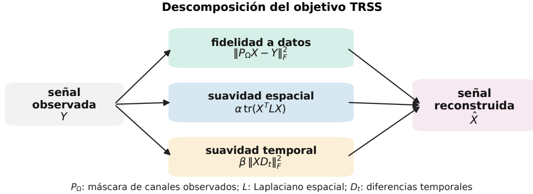
Figura 2.3: Descomposición del operador TRSS. La reconstrucción combina fidelidad a los canales observados, suavidad espacial inducida por el Laplaciano del grafo y suavidad temporal inducida por diferencias finitas. El término temporal no agrega información externa: restringe el espacio de soluciones admisibles mediante D_t .
