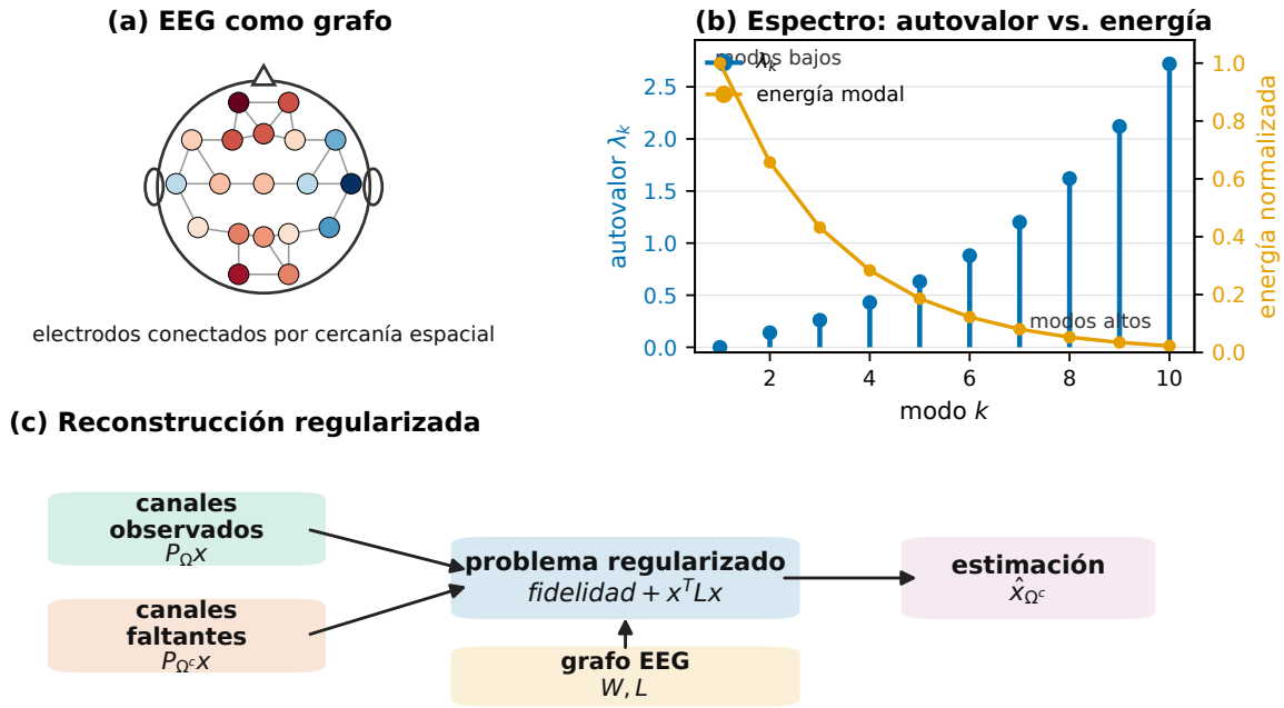
Figura 2.2: Conceptos fundamentales de GSP aplicados a EEG. (a) Los electrodos forman un grafo ponderado sobre una topografía de cabeza; las aristas codifican cercanía espacial. (b) El espectro del Laplaciano ordena los modos desde variación suave hasta variación rápida. La curva azul muestra autovalores, mientras que la curva naranja ilustra que la energía de una señal suave tiende a concentrarse en modos bajos. (c) La reconstrucción regularizada estima los canales faltantes combinando fidelidad a los canales observados y suavidad inducida por el grafo.
