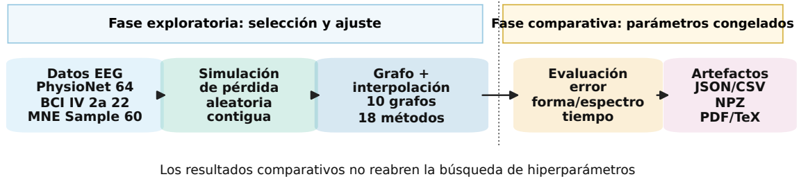
Figura 3.2: Diagrama de bloques de la arquitectura del sistema experimental. Cinco módulos con interfaces explícitas operan en cadena. La figura distingue fase exploratoria y fase comparativa, indicando que los resultados comparativos no reabren la búsqueda de hiperparámetros.
