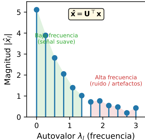
(c) Transformada de Fourier en Grafos (GFT)
