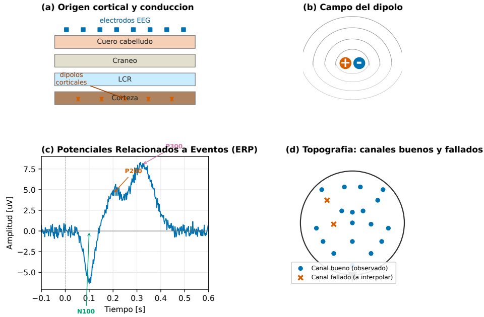
Figura 2.1: Generación de la señal EEG por poblaciones neuronales corticales y su propagación hasta los electrodos de superficie. La conducción volumétrica a través del cráneo actúa como un filtro espacial paso-bajo. Adaptado de [18].
