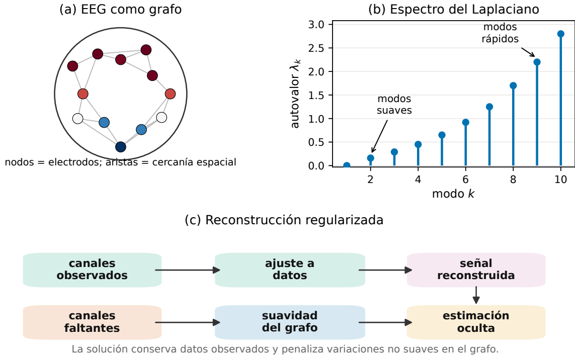
Figura 2.2: Conceptos fundamentales de GSP aplicados a EEG. (a) Los electrodos forman un grafo ponderado; (b) el espectro del Laplaciano ordena los modos desde variación suave hasta variación rápida; (c) la reconstrucción regularizada combina fidelidad a los canales observados con penalización de variación sobre el grafo.
