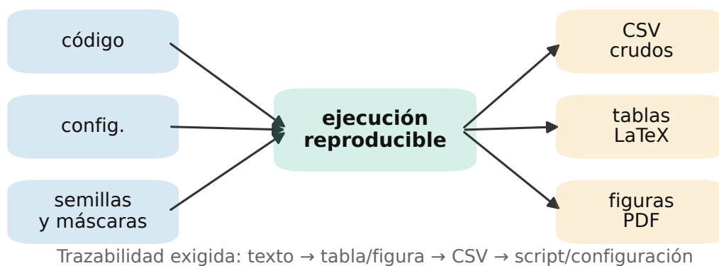
Figura 3.3: Cadena de trazabilidad experimental. Cada afirmación cuantitativa puede rastrearse desde el texto hasta una tabla o figura, desde allí al archivo CSV correspondiente y finalmente al script que generó el resultado.
