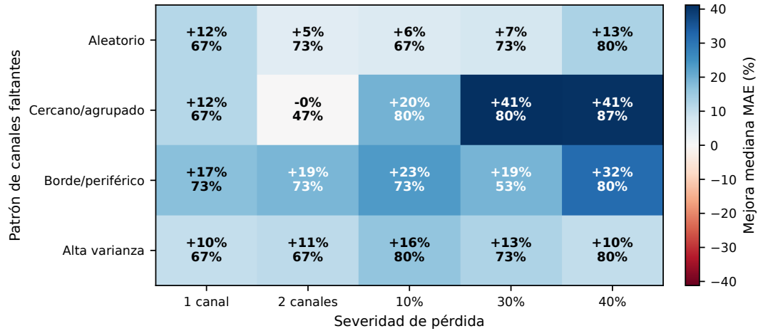
Figura 6.6: Mapa de calor de mejora mediana de MAE para TRSS fijo frente a MNE. Cada celda muestra la mejora mediana y, debajo, la tasa de victoria. La ventaja crece cuando la pérdida elimina información espacial local, especialmente en patrones cercanos o periféricos de alta severidad.
