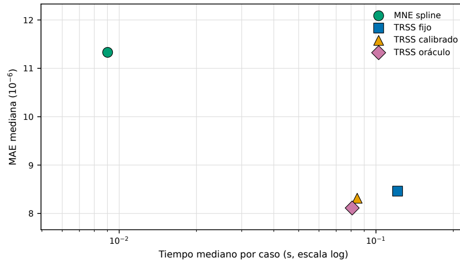
Figura 6.1: Compromiso entre precisión y tiempo de cómputo en la evaluación confirmatoria. TRSS desplaza el MAE hacia valores menores, pero se ubica a la derecha de MNE en la escala logarítmica de tiempo, lo que evidencia el costo computacional de la regularización temporal.
