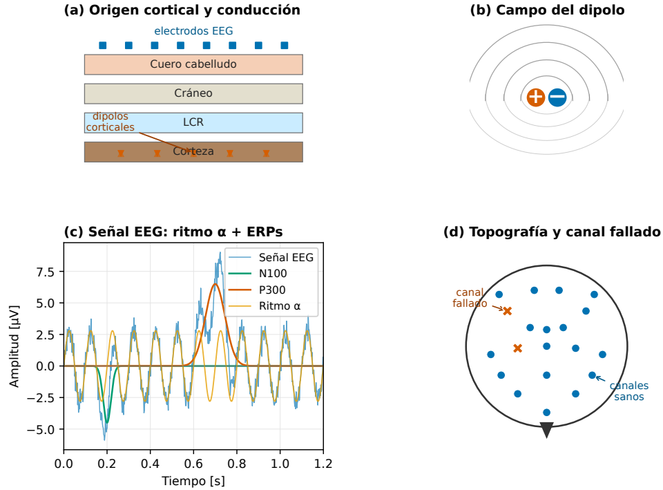
Figura 2.1: Generación de la señal EEG por poblaciones neuronales corticales y su propagación hasta los electrodos de superficie. La conducción volumétrica a través del cráneo actúa como un filtro espacial paso-bajo. Adaptado de [17].
