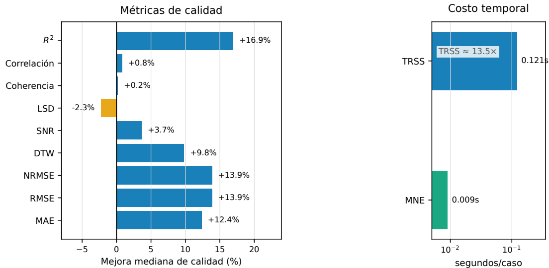
Figura 6.2: Portafolio visual de métricas para TRSS fijo frente a MNE. El panel izquierdo muestra métricas de calidad con valores positivos favorables a TRSS y negativos favorables a MNE; el panel derecho separa el costo temporal para que la diferencia de escala no comprima las métricas de precisión.
