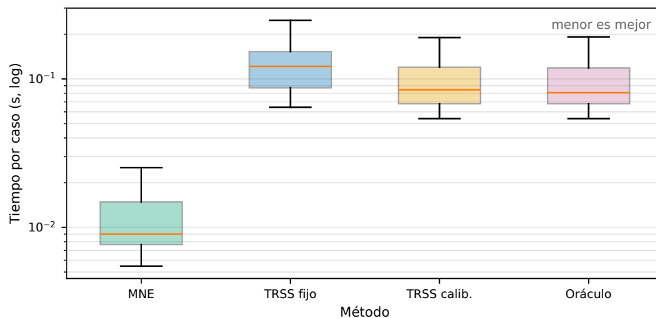
Figura 6.10: Distribución de tiempos por caso en la evaluación confirmatoria. La diferencia de costo es consistente: TRSS mejora varias métricas de reconstrucción, pero MNE conserva una ventaja clara en velocidad.
