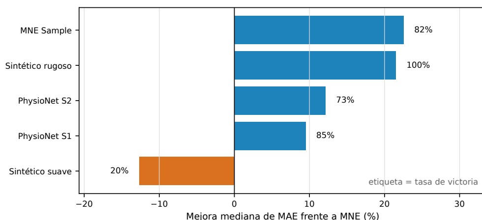
Figura 6.5: Mejora mediana de MAE de TRSS fijo frente a MNE por conjunto de datos. La señal sintética suave actúa como control negativo: cuando se cumple fuertemente el supuesto de suavidad espacial, MNE puede ser superior.
