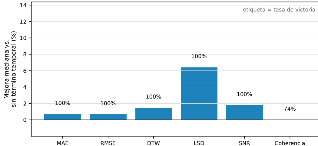
Figura 6.7: Ablación del componente temporal: mejora mediana de TRSS completo frente a TRSS sin término temporal. La contribución temporal es consistente dentro de la familia TRSS, aunque su magnitud es menor que las diferencias entre familias de métodos.
