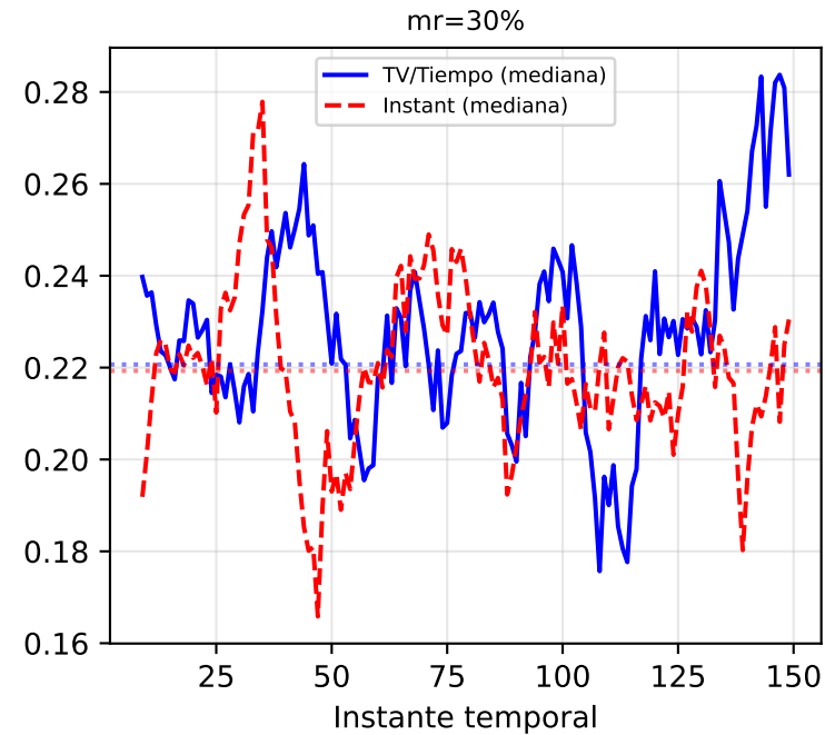
it06b_kalofolias_nnk_3syn — Error de Reconstrucción Temporal por Escenario
