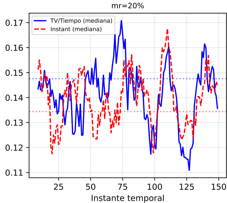
it07b_knn_3syn — Error de Reconstrucción Temporal por Escenario
