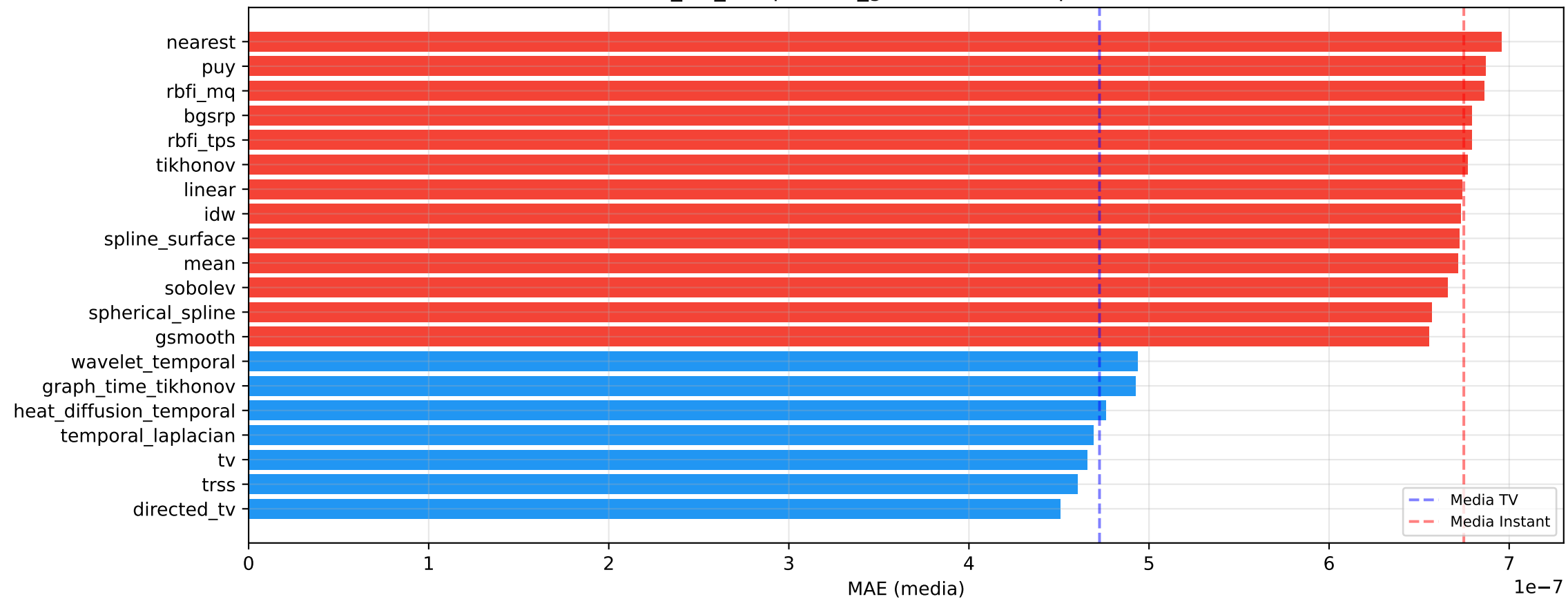
it66_bci_competition_gaussian — MAE por Método
