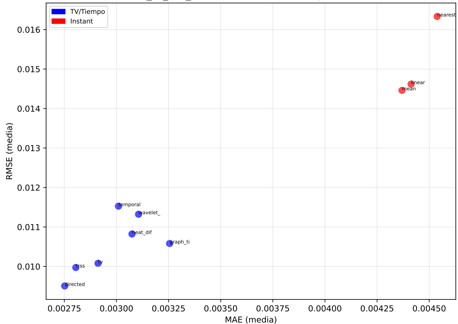
it70_all_five_datasets — MAE vs RMSE por Método
