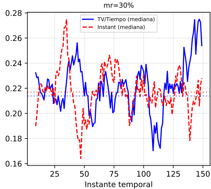
it09_tikhonov_rbf_focus — Error de Reconstrucción Temporal por Escenario
