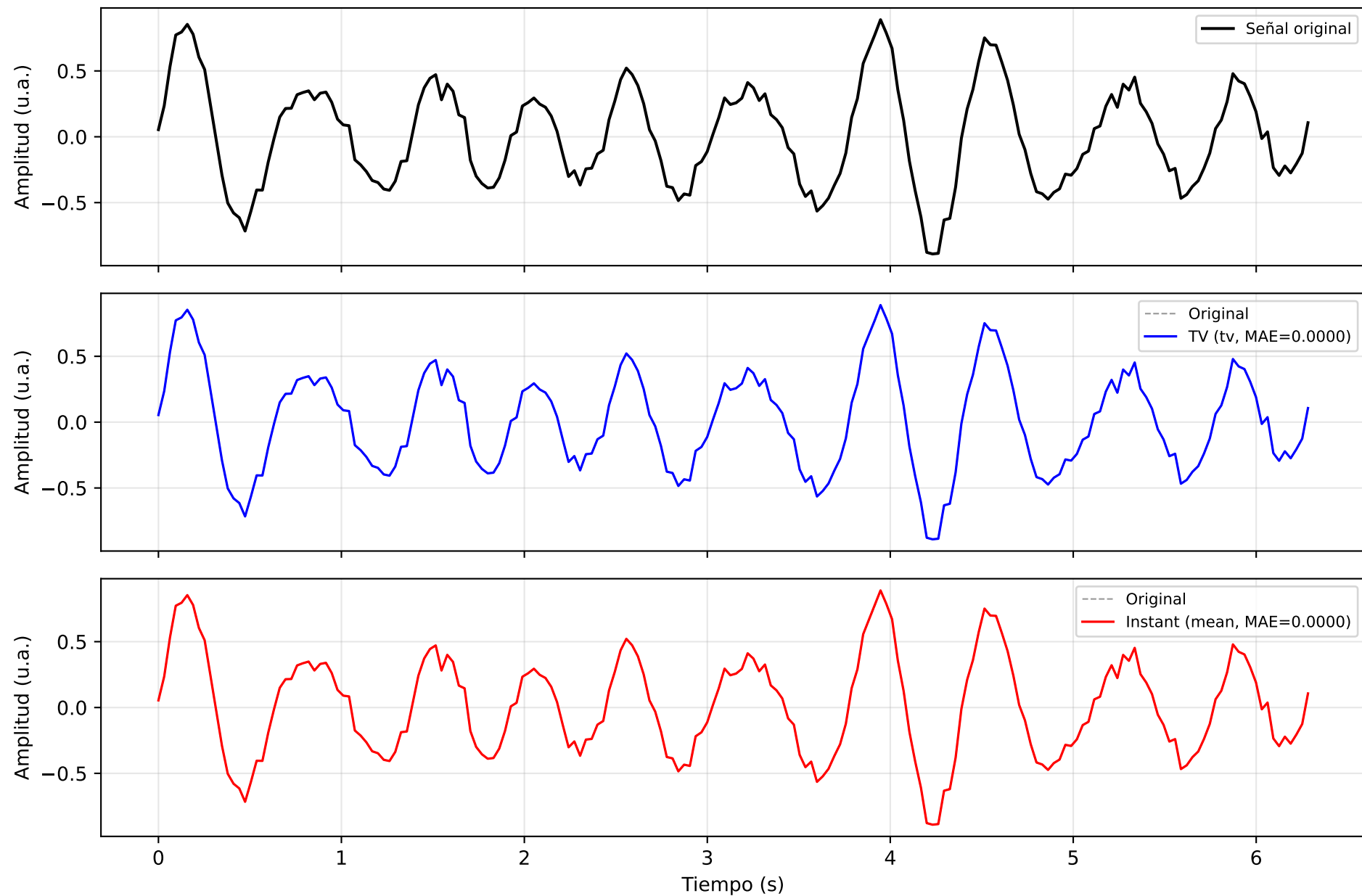
it11_physionet_high_missing — Señal EEG: Original vs Reconstrucción
