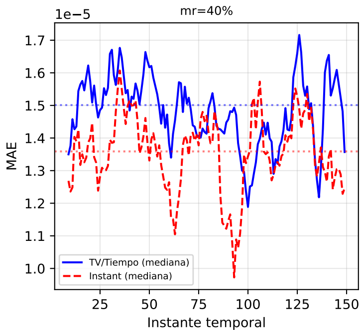
it11_physionet_high_missing — Error de Reconstrucción Temporal por Escenario
