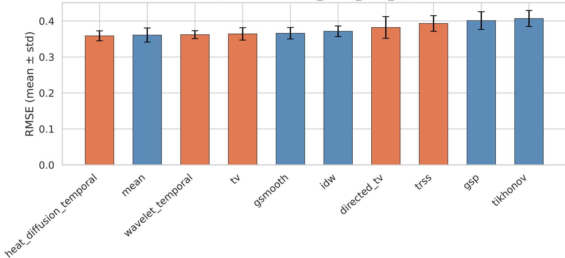
Top-10 RMSE — it12_vknng_knng_3syn
