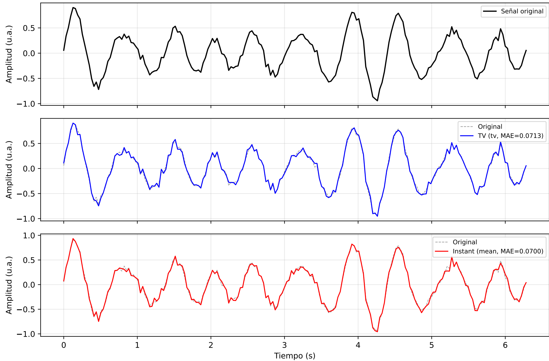
it14_low_missing_synthetic — Señal EEG: Original vs Reconstrucción
