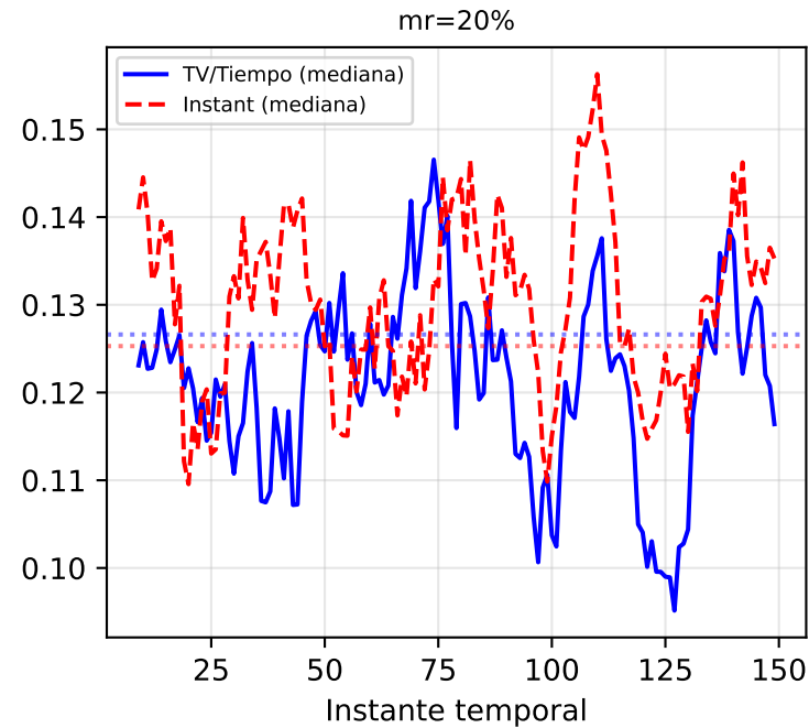
it17_synthetic_broad_all_graphs — Error de Reconstrucción Temporal por Escenario
