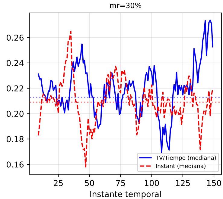
it17_synthetic_broad_all_graphs — Error de Reconstrucción Temporal por Escenario
