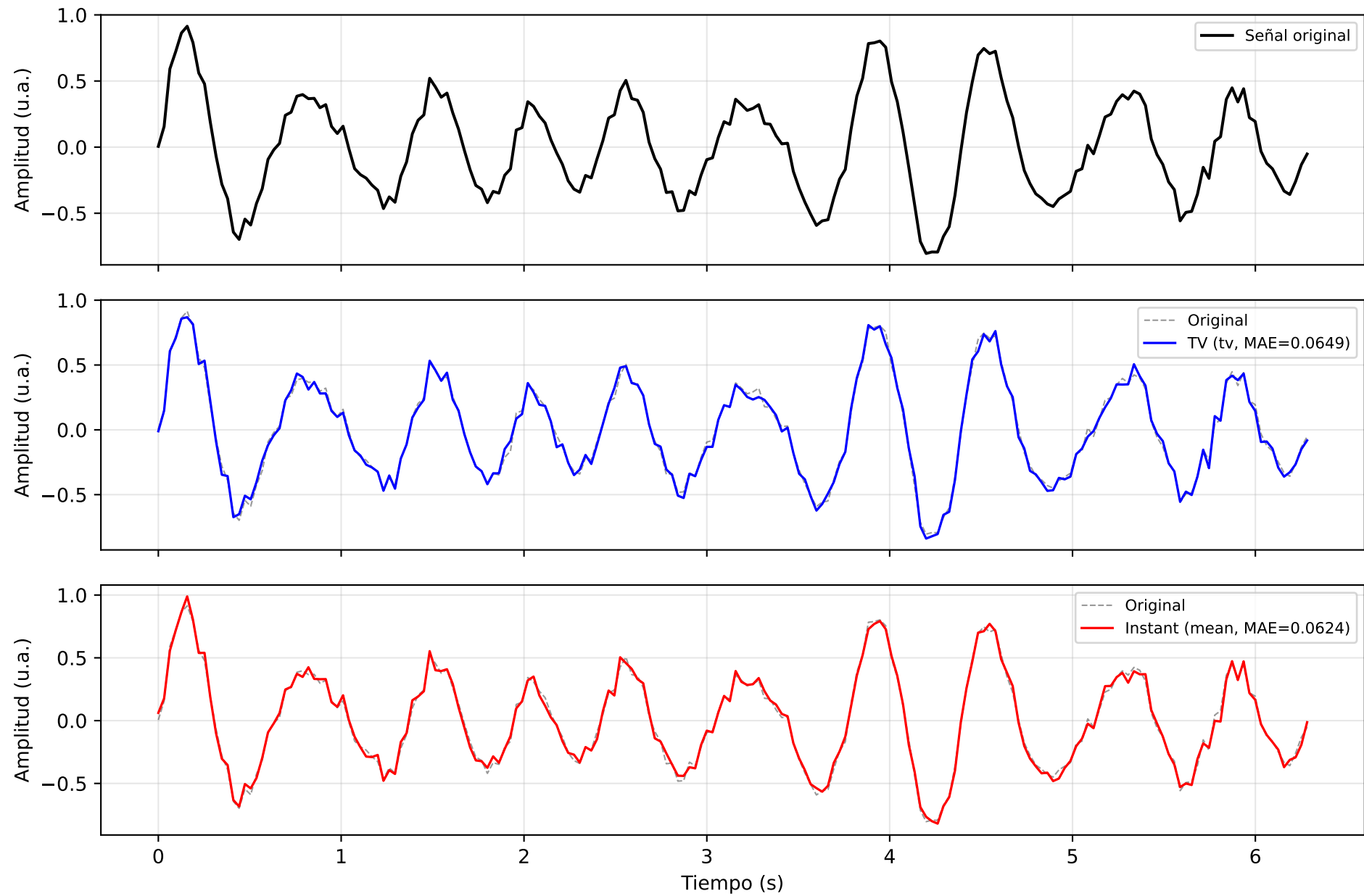
it25_alpha_beta_two_bands — Señal EEG: Original vs Reconstrucción
