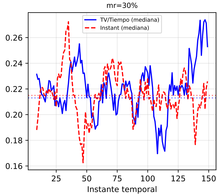
it30_knn_k5_3syn — Error de Reconstrucción Temporal por Escenario
