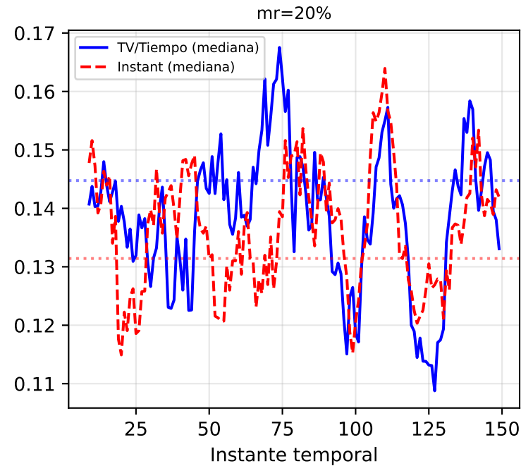
it35_all4_kalofolias — Error de Reconstrucción Temporal por Escenario
