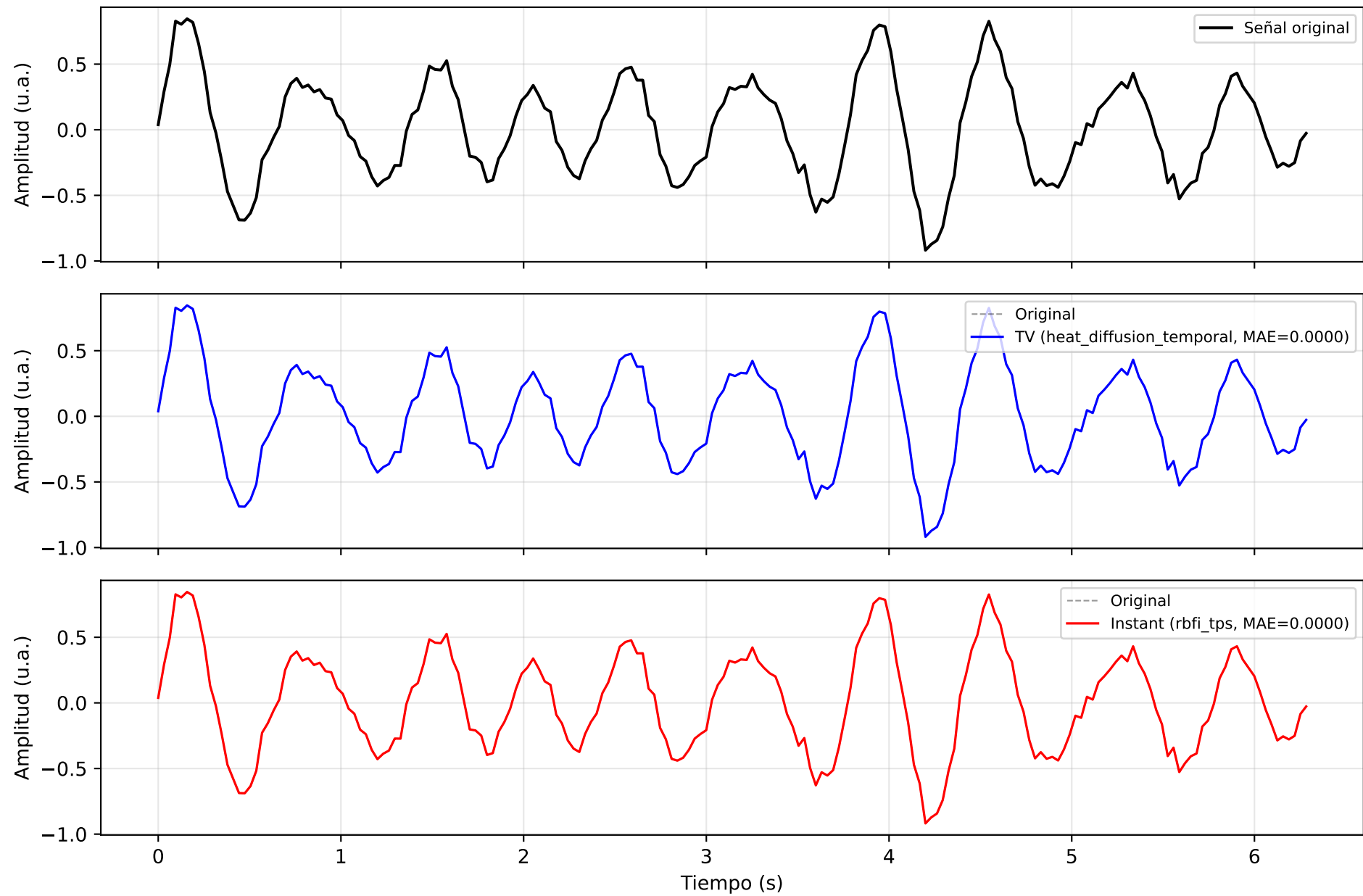
it46_physionet_multisubj_kalofolias — Señal EEG: Original vs Reconstrucción
