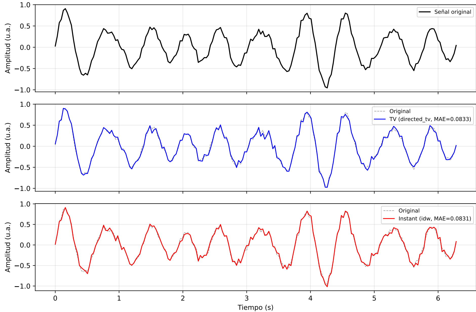
it58_broad_low_missing — Señal EEG: Original vs Reconstrucción
