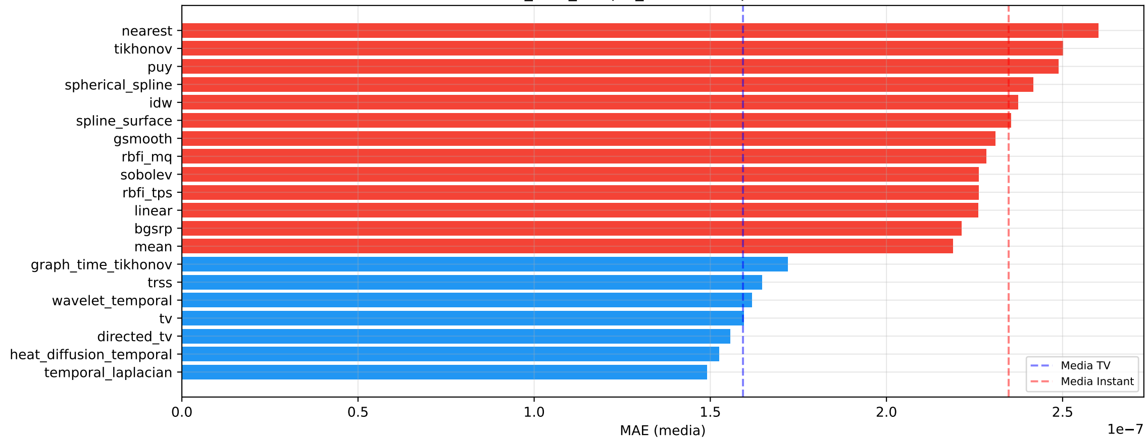
it61_mne_sample_knn — MAE por Método
