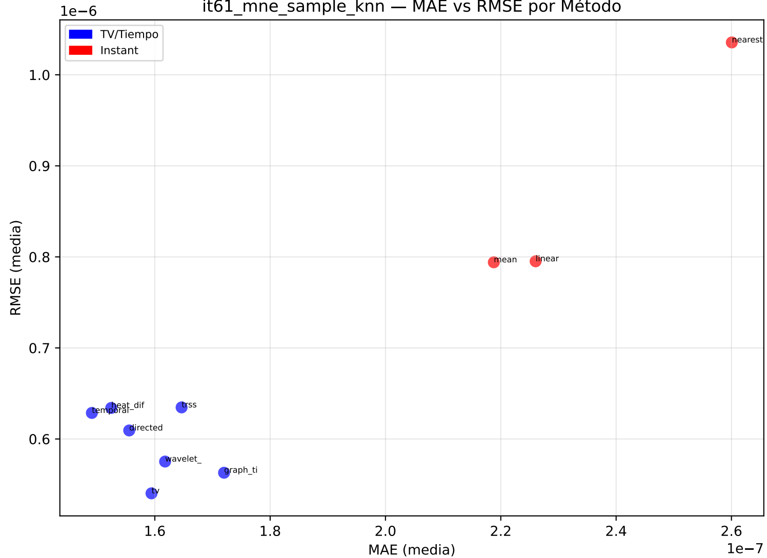
it61_mne_sample_knn — MAE vs RMSE por Método
