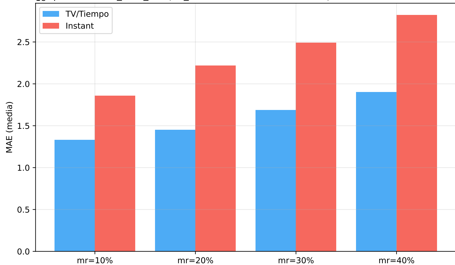
1e-7 it61_mne_sample_knn — Familia TV vs Instant por Escenario
