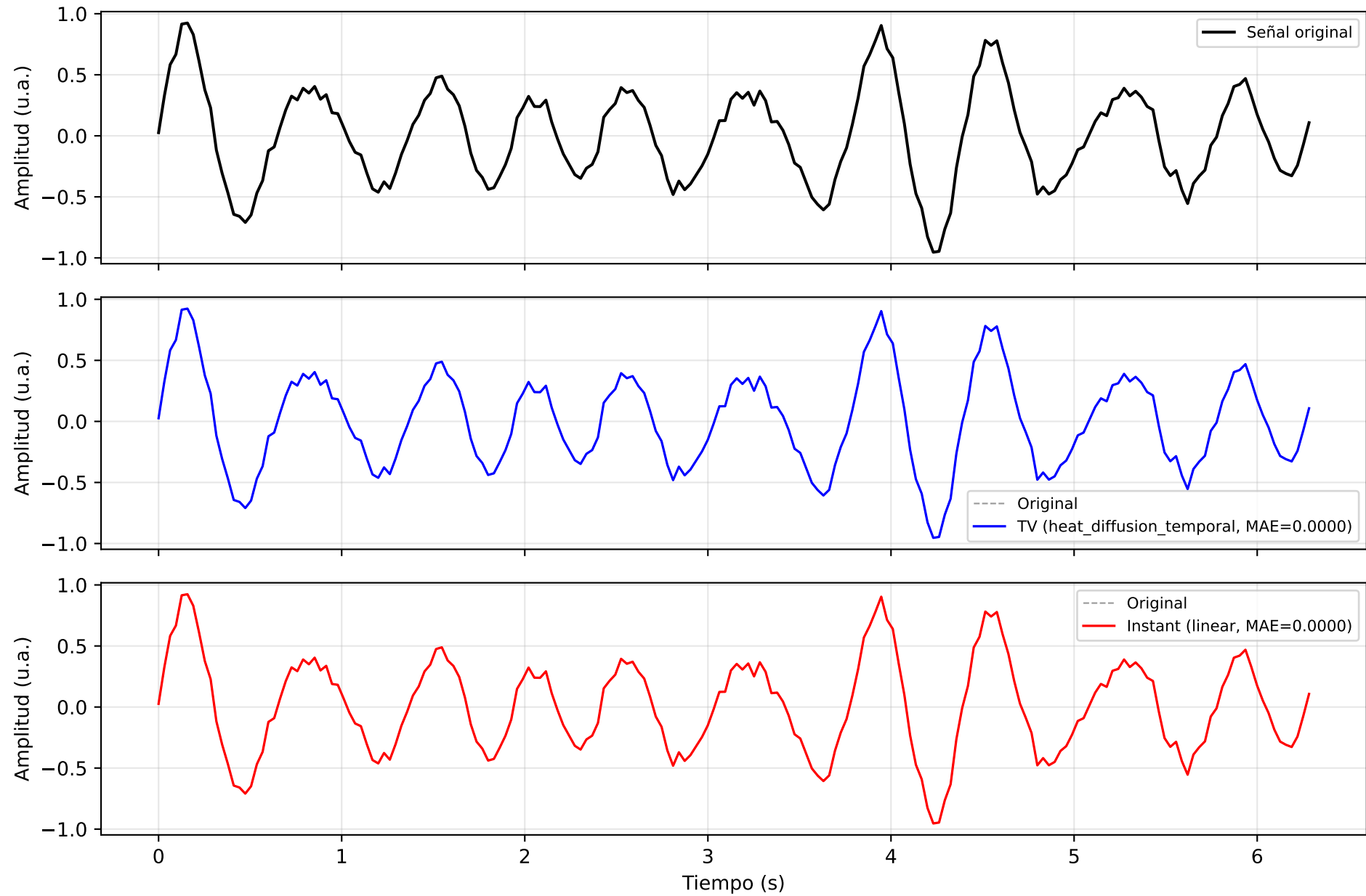
it61_mne_sample_knn — Señal EEG: Original vs Reconstrucción
