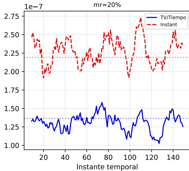
it61_mne_sample_knn — Error de Reconstrucción Temporal por Escenario
