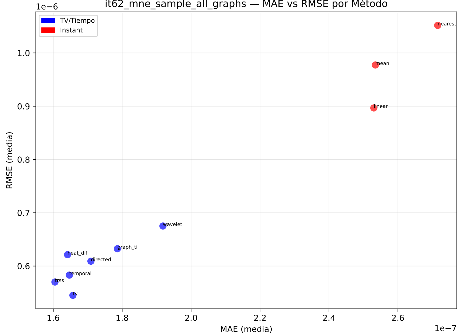
it62_mne_sample_all_graphs — MAE vs RMSE por Método
