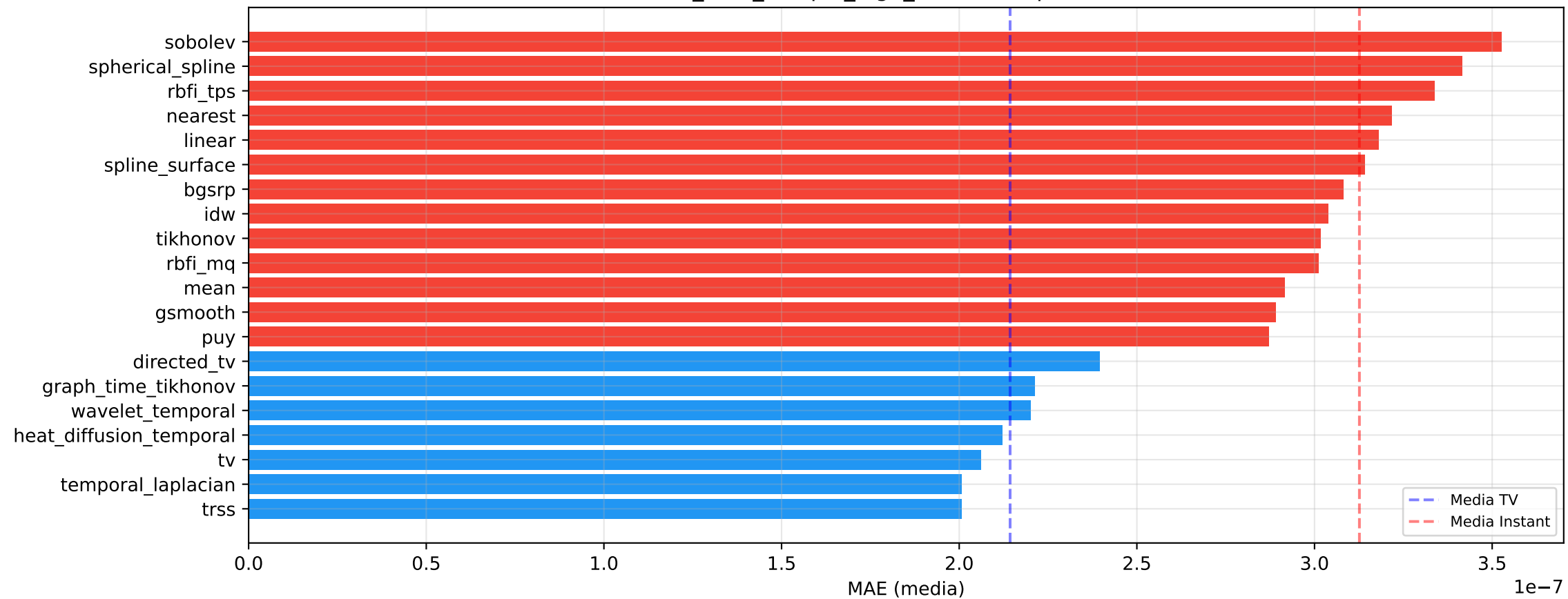
it63_mne_sample_high_mr — MAE por Método
