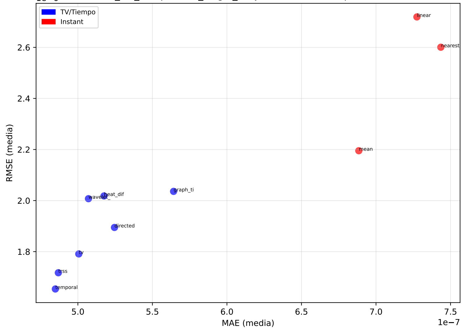
it64_bci_competition_single_subj — MAE vs RMSE por Método
