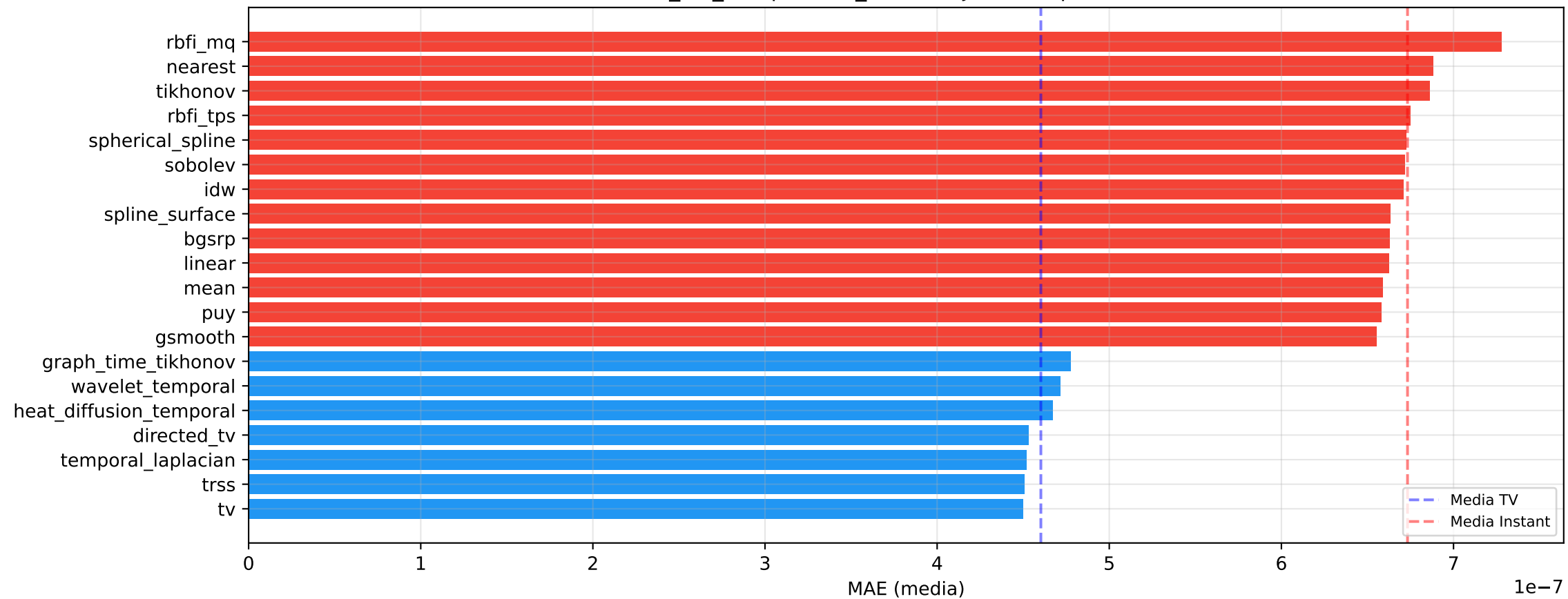
it65_bci_competition_multisubj — MAE por Método
