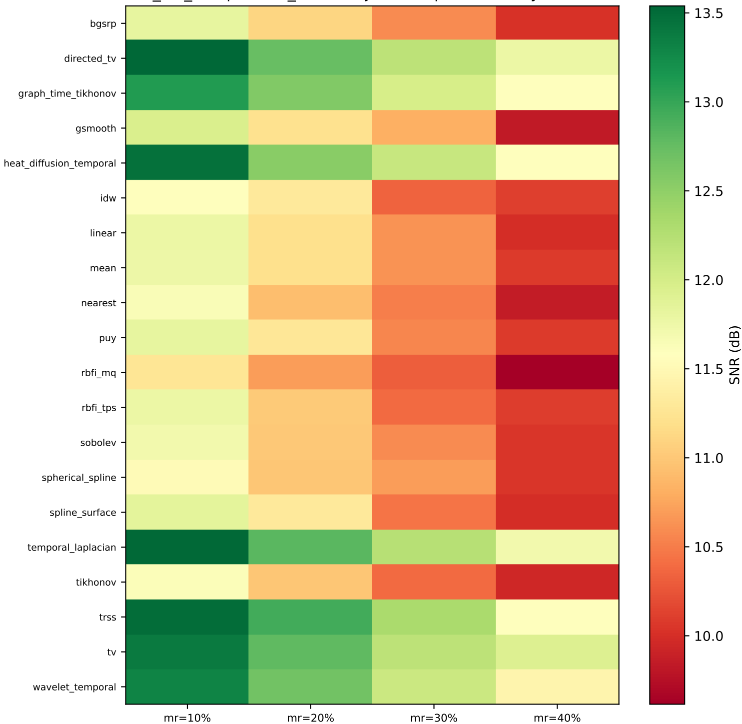
it65_bci_competition_multisubj — SNR por Método y Escenario
