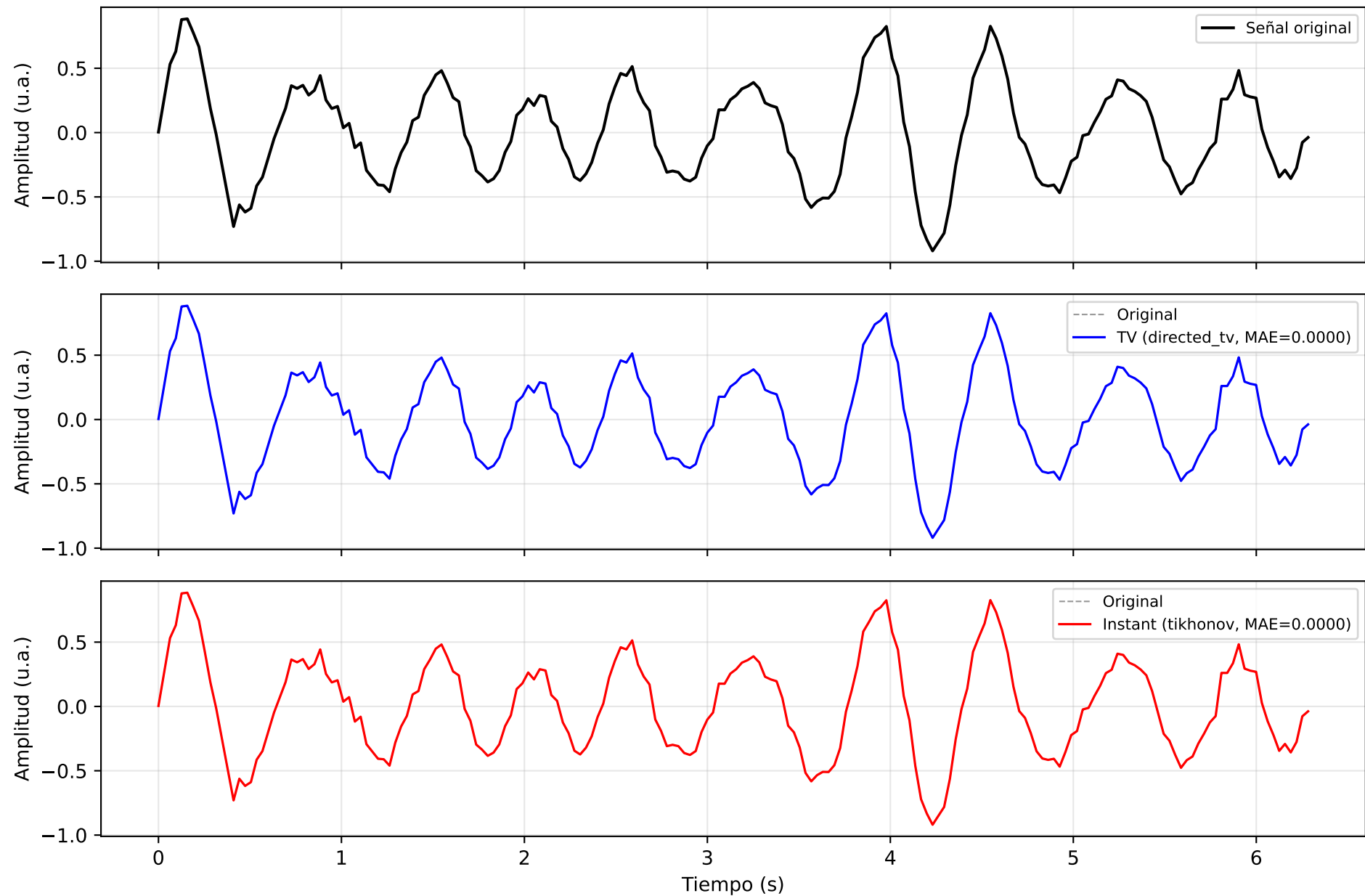
it66_bci_competition_gaussian — Señal EEG: Original vs Reconstrucción
