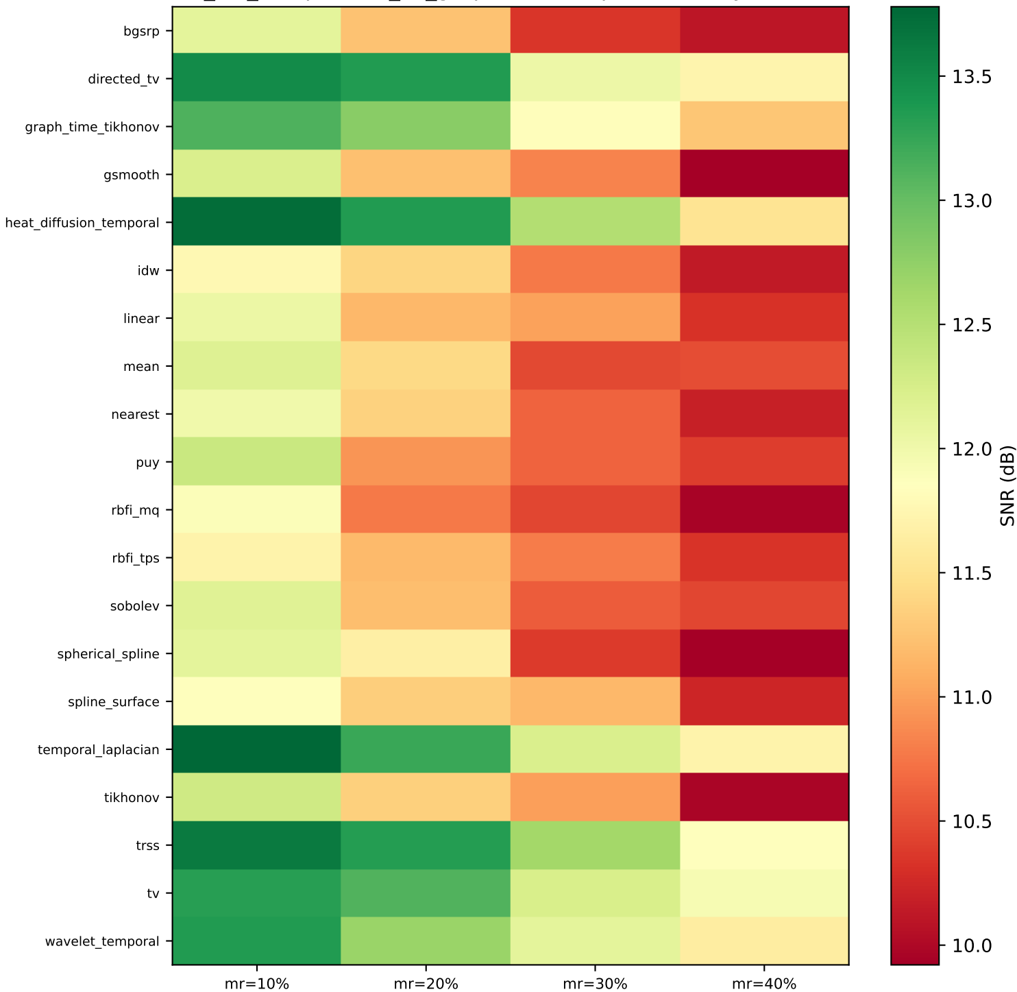
it67_bci_competition_all_graphs — SNR por Método y Escenario
