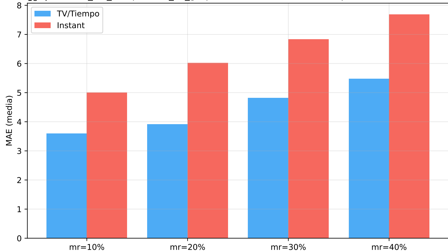
1e-7 it67_bci_competition_all_graphs — Familia TV vs Instant por Escenario
