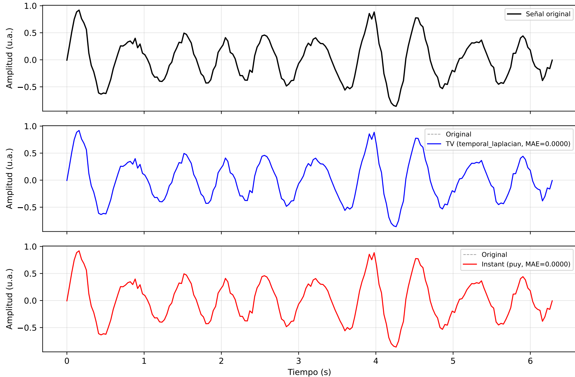
it67_bci_competition_all_graphs — Señal EEG: Original vs Reconstrucción
