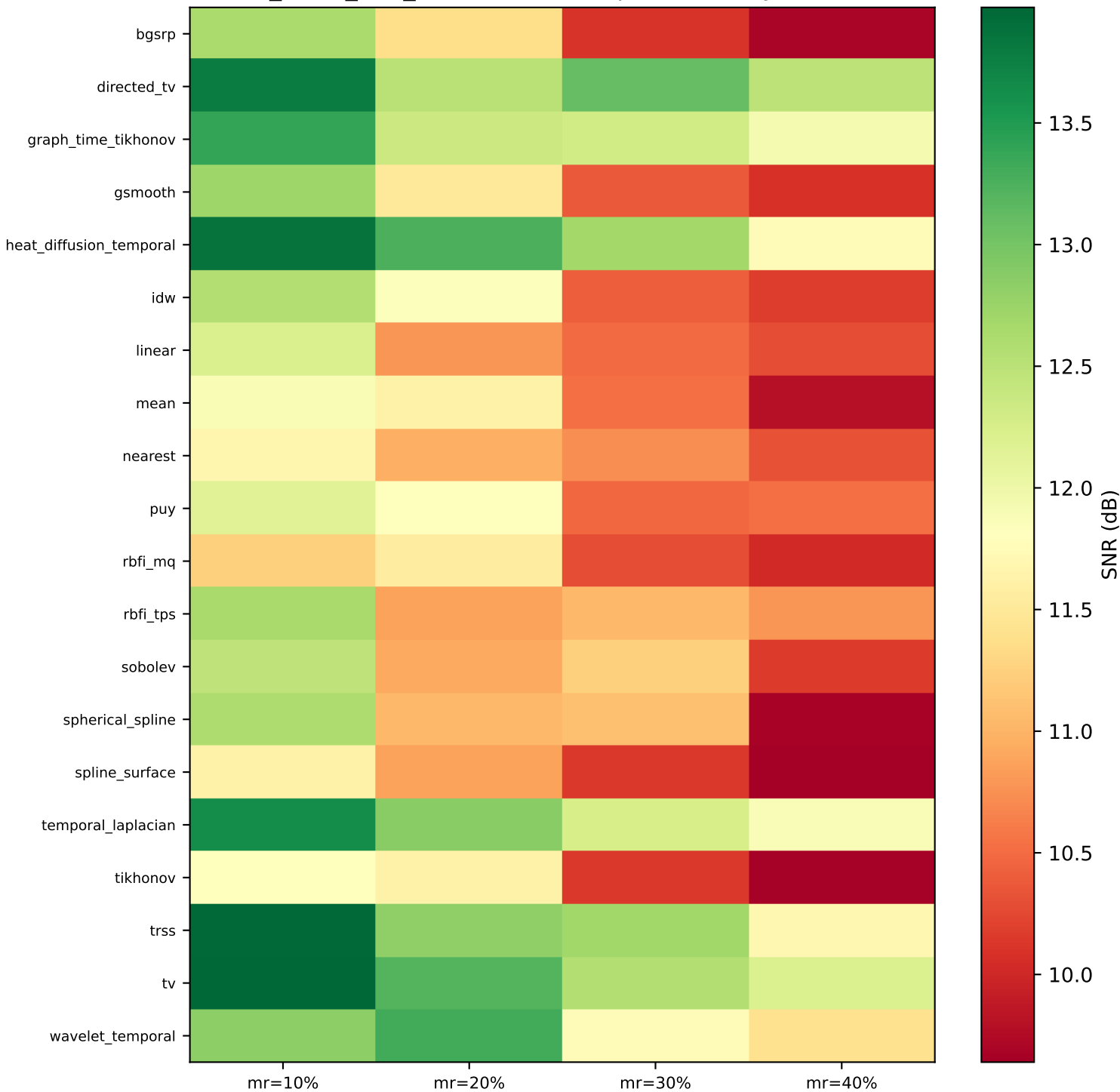
it68_three_real_datasets — SNR por Método y Escenario
