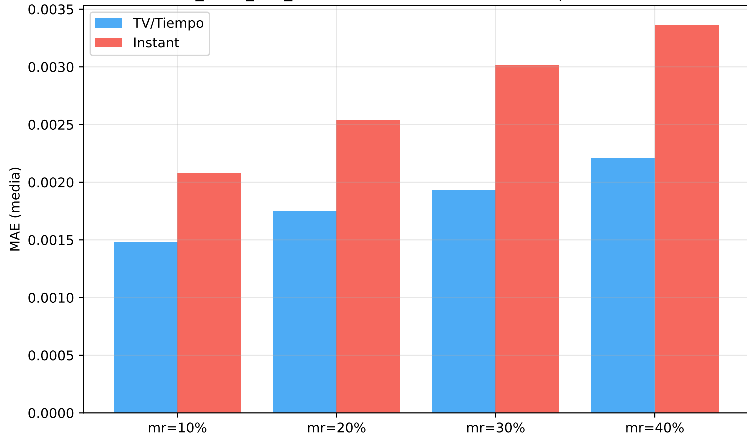
it68_three_real_datasets — Familia TV vs Instant por Escenario
