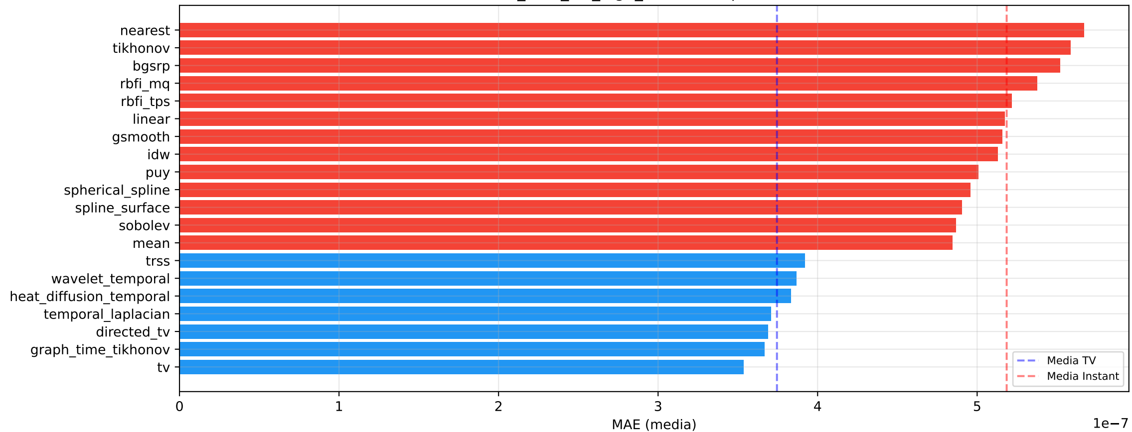
it69_mne_bci_high_mr — MAE por Método
