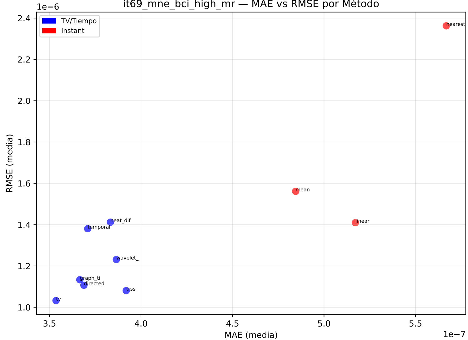
it69_mne_bci_high_mr — MAE vs RMSE por Método
