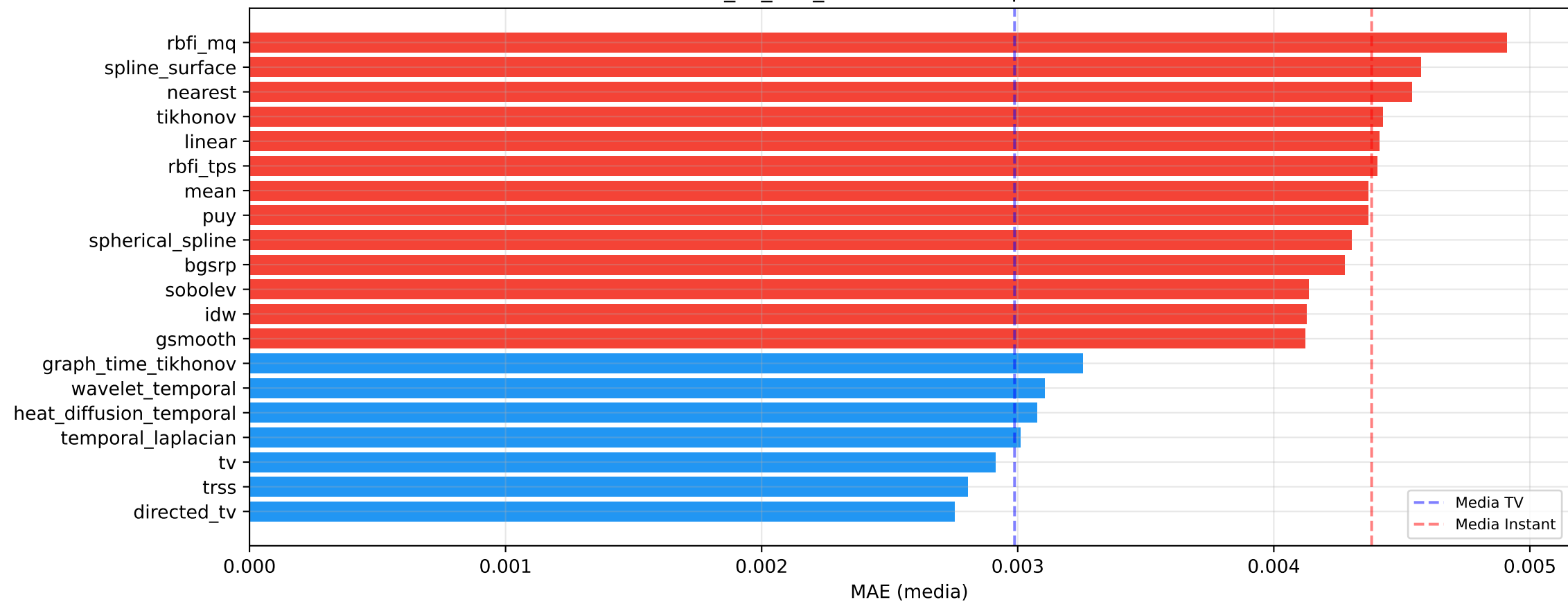
it70_all_five_datasets — MAE por Método
