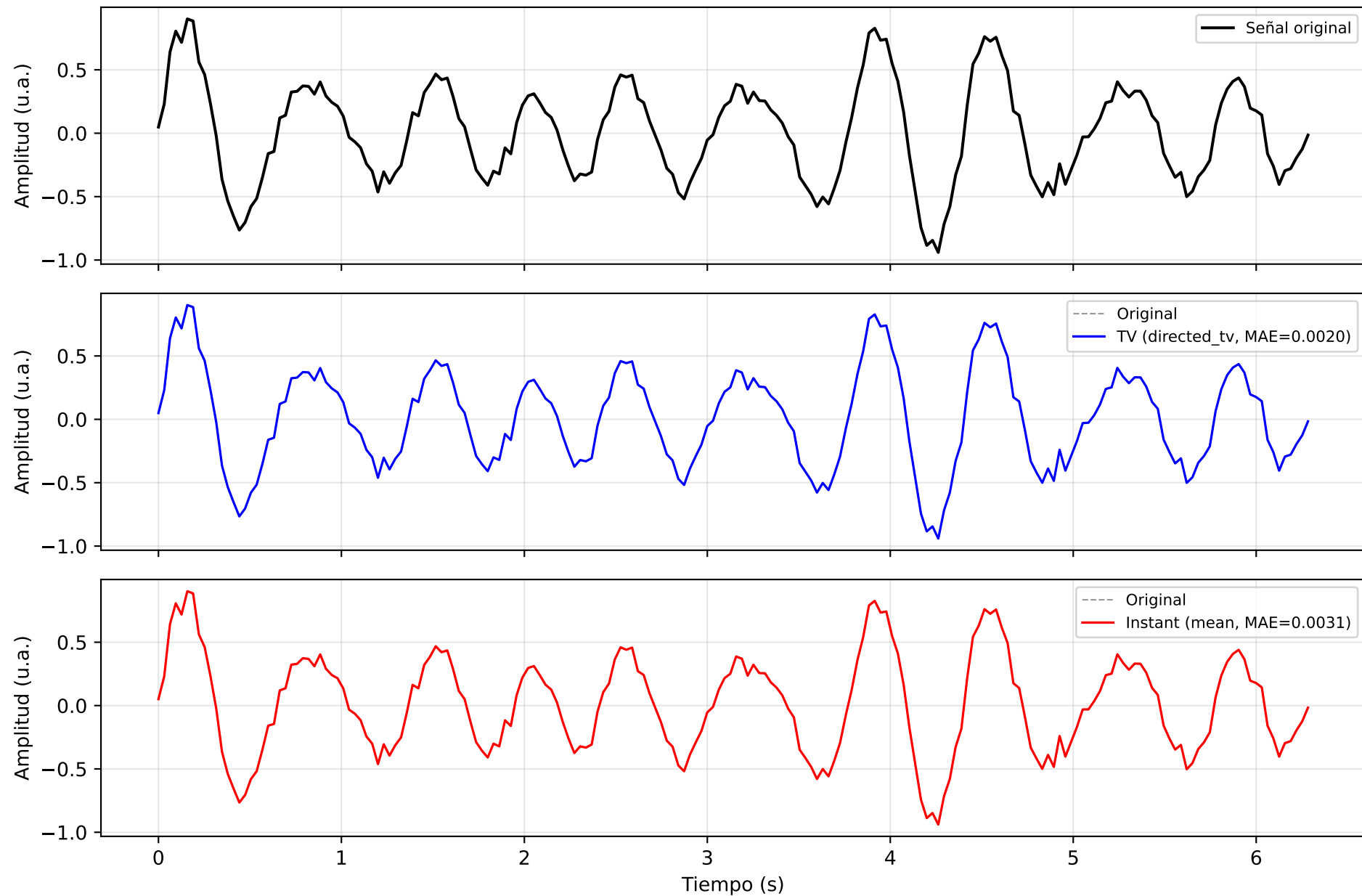
it70_all_five_datasets — Señal EEG: Original vs Reconstrucción
