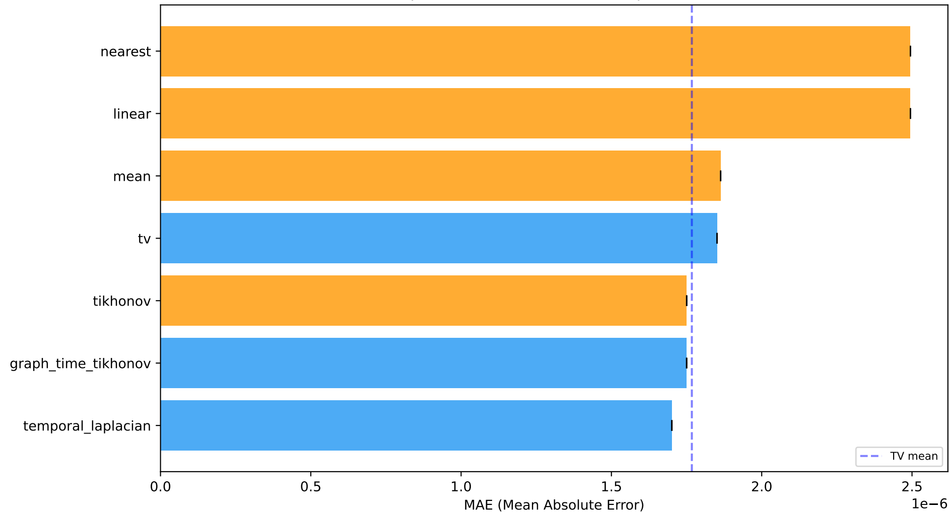
it74_few_missing_2ch_mne_proxy MAE por Método (azul=TV, naranja=Instante)
