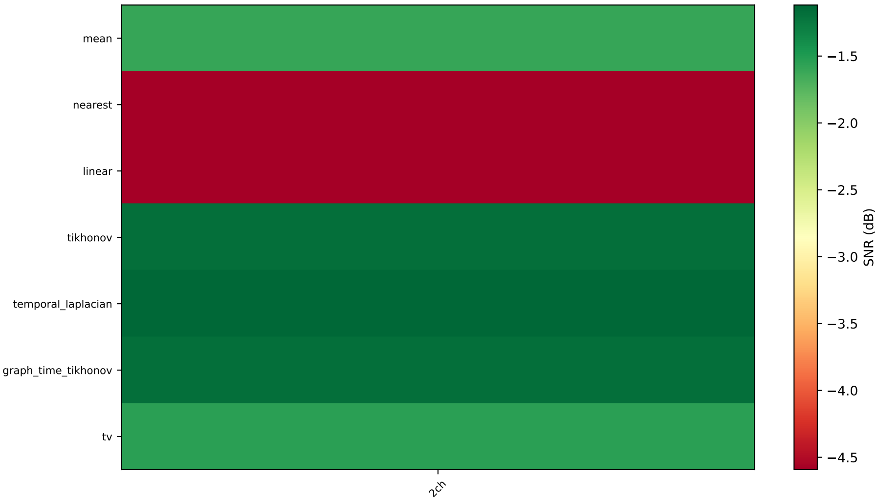
it74_few_missing_2ch_mne_proxy SNR (dB): Métodos × Escenarios
