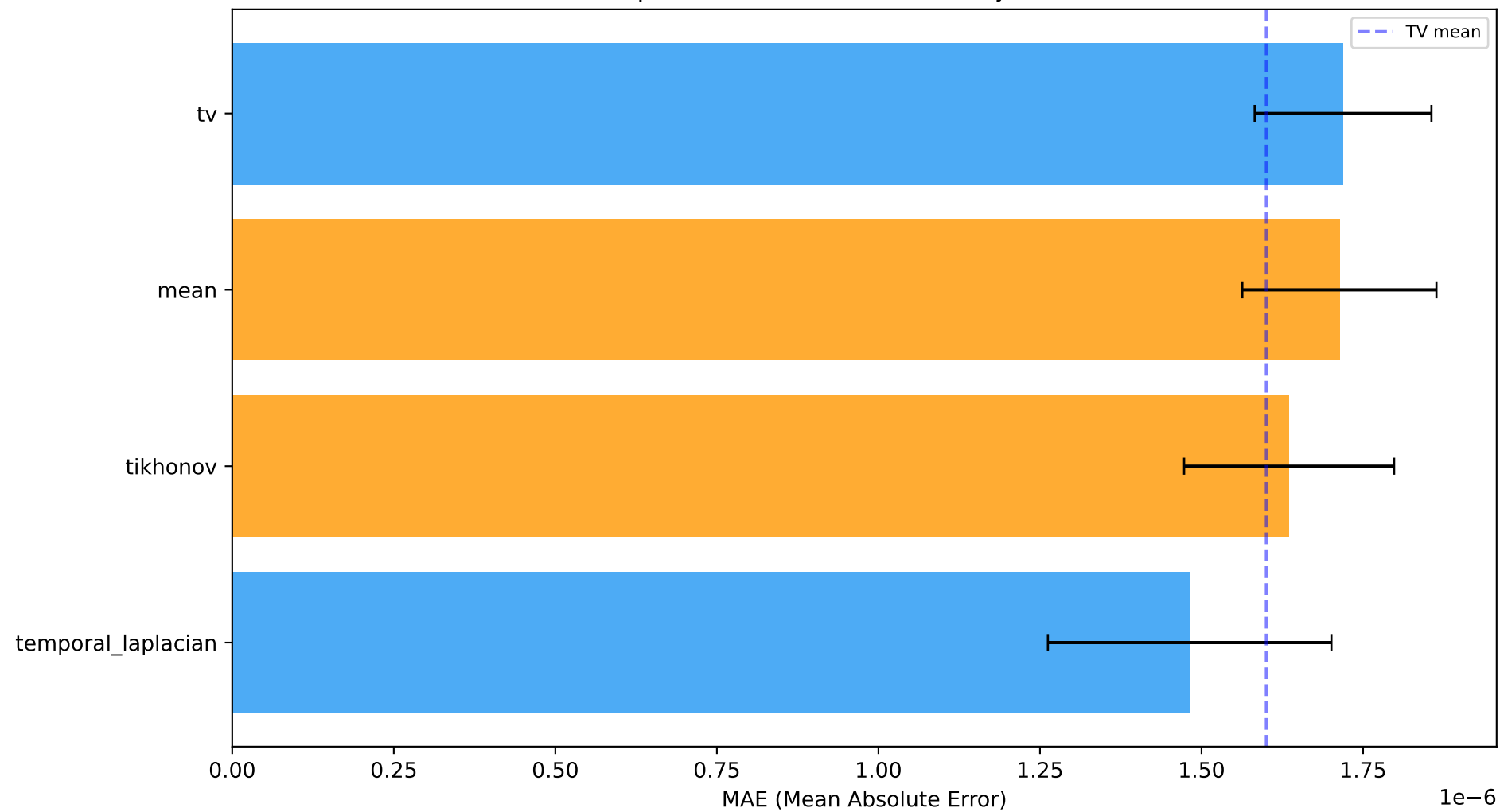
it76_few_missing_mne_all_graphs MAE por Método (azul=TV, naranja=Instante)
