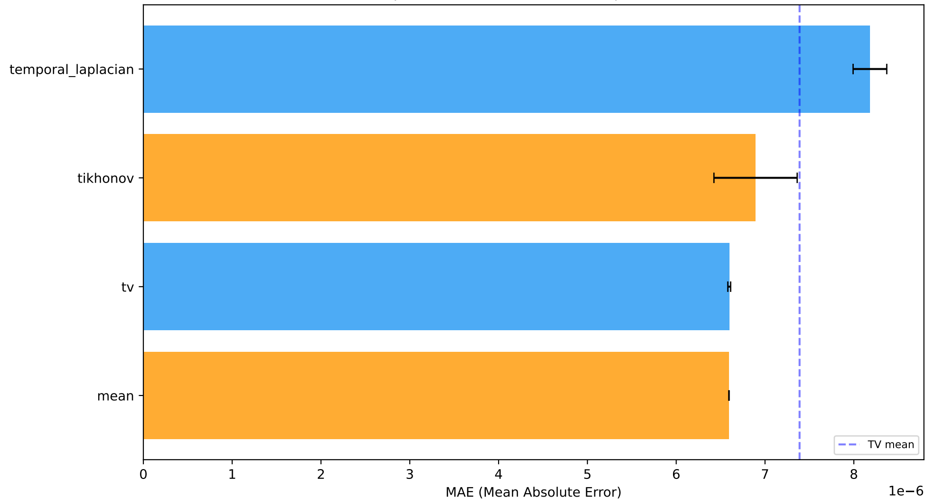
it77_few_missing_bci_all_graphs MAE por Método (azul=TV, naranja=Instante)
