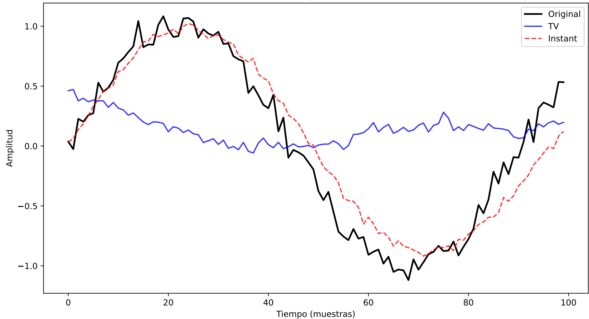
it78_few_missing_1ch_tv_focus Reconstrucción: Original vs TV vs Instante
