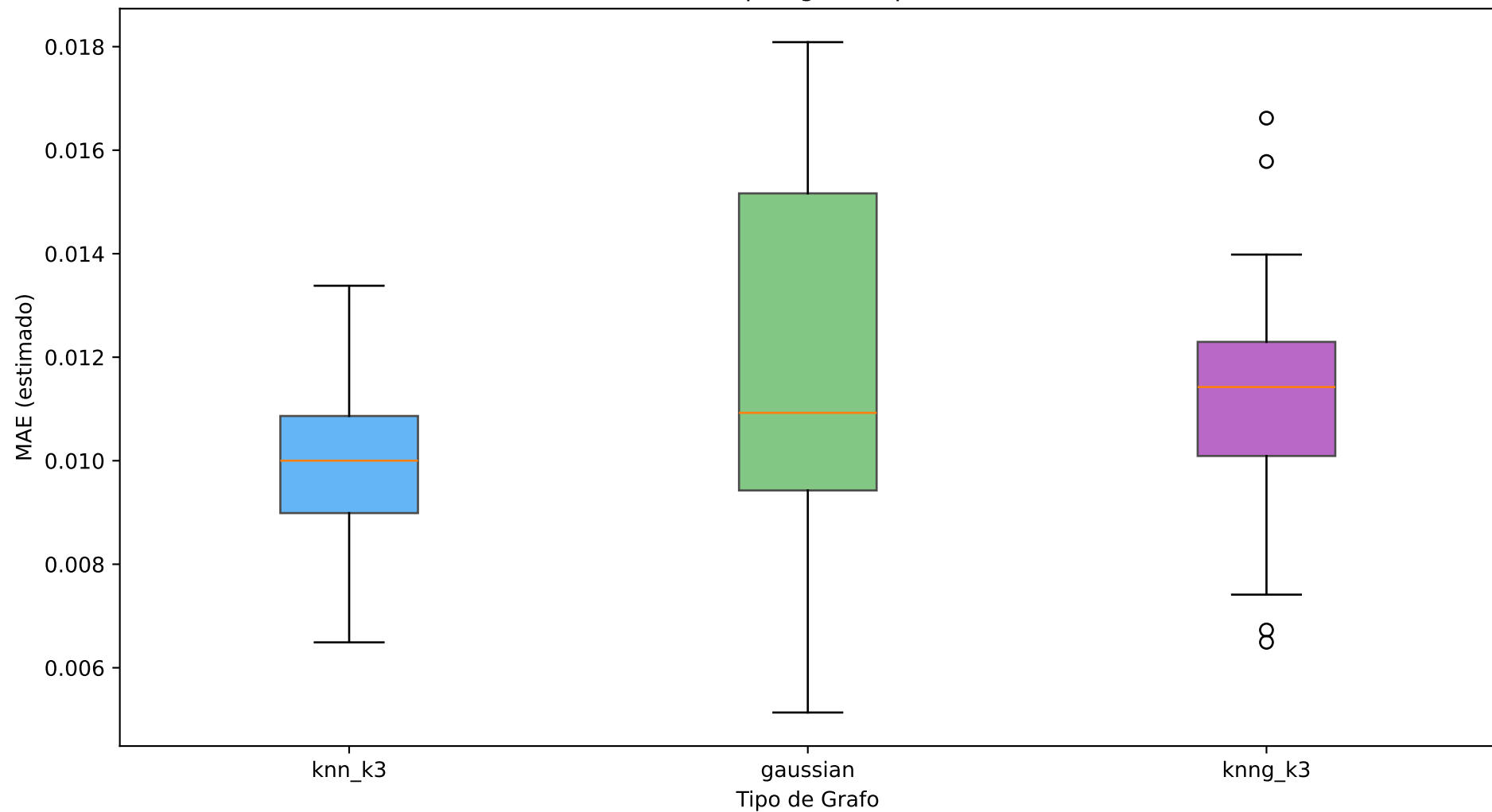
it79_few_missing_2ch_tv_focus Influencia Topología (esquemático)
