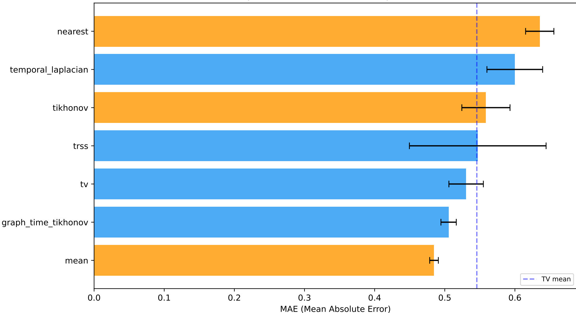
it82_full_signal_recon_synthetic MAE por Método (azul=TV, naranja=Instante)
