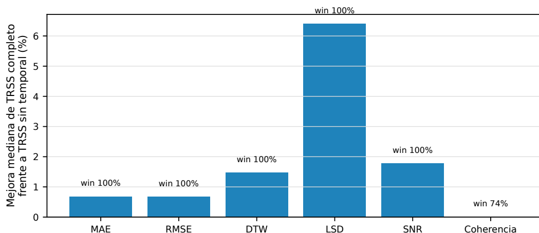
Figura 6.5: Ablación del componente temporal: mejora mediana de TRSS completo frente a TRSS sin término temporal. La contribución temporal es consistente dentro de la familia TRSS, aunque su magnitud es menor que las diferencias entre familias de métodos.
