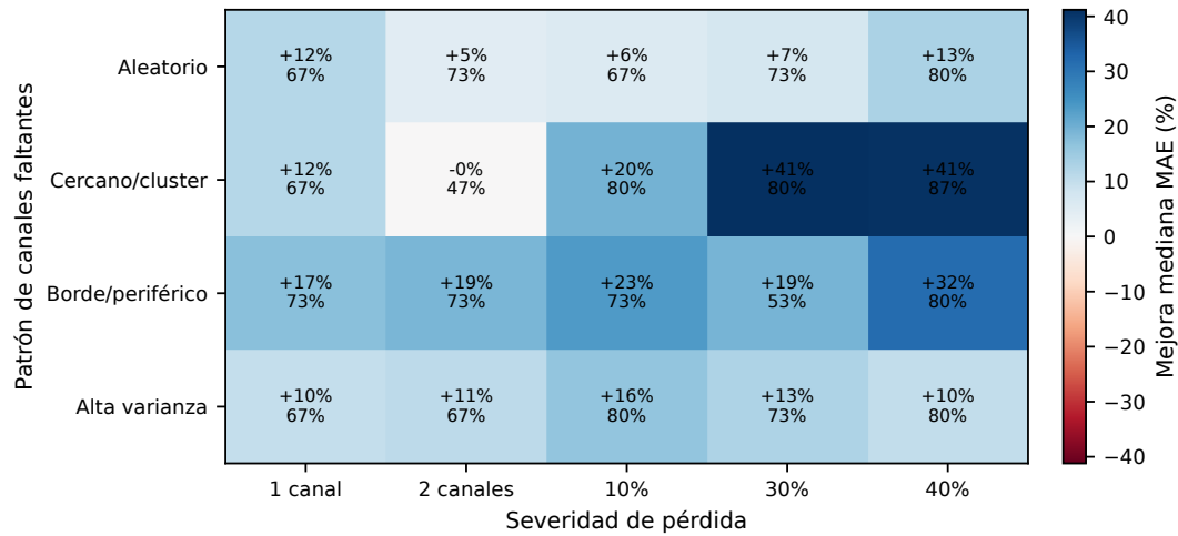
Figura 6.4: Mapa de calor de mejora mediana de MAE para TRSS fijo frente a MNE. Cada celda muestra la mejora mediana y, debajo, la tasa de victoria. La ventaja crece cuando la pérdida elimina información espacial local, especialmente en patrones cercanos o periféricos de alta severidad.
