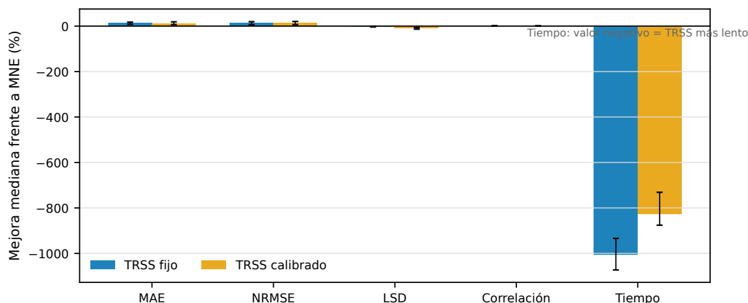
Figura 6.2: Mejoras medianas de TRSS frente a MNE con intervalos bootstrap al 95 %. Las barras positivas favorecen a TRSS; las barras negativas favorecen a MNE o indican mayor tiempo de ejecución de TRSS. El gráfico muestra simultáneamente la ganancia en MAE/NRMSE y las dos advertencias principales: LSD y costo temporal.
