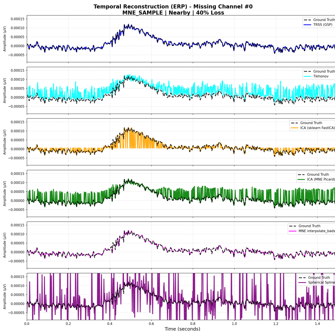
Figura 6.6: Ejemplo cualitativo de reconstrucción temporal bajo pérdida cercana severa. La figura ilustra la diferencia morfológica que las métricas agregadas capturan de forma resumida.
