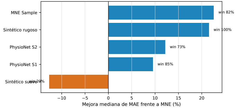
Figura 6.3: Mejora mediana de MAE de TRSS fijo frente a MNE por conjunto de datos. La señal sintética suave actúa como control negativo: cuando se cumple fuertemente el supuesto de suavidad espacial, MNE puede ser superior.
