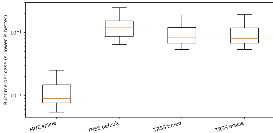
Figura 6.8: Distribución de tiempos por caso en la evaluación confirmatoria. La diferencia de costo es consistente: TRSS mejora varias métricas de reconstrucción, pero MNE conserva una ventaja clara en velocidad.
