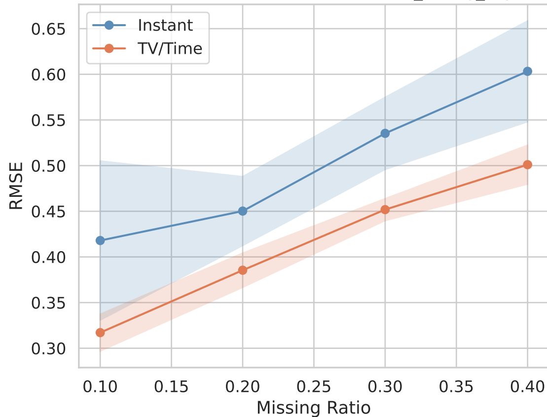
RMSE — TV/Time vs Instant — it16b_vknng_3syn
