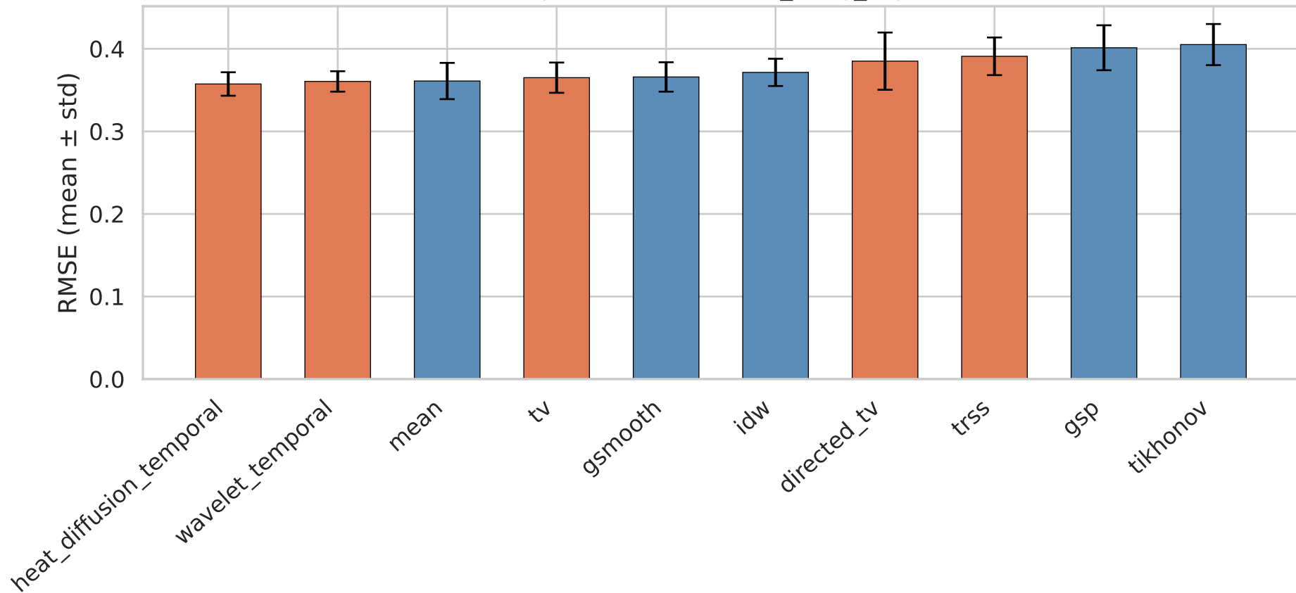
Top-10 RMSE — it23b_knng_3syn
