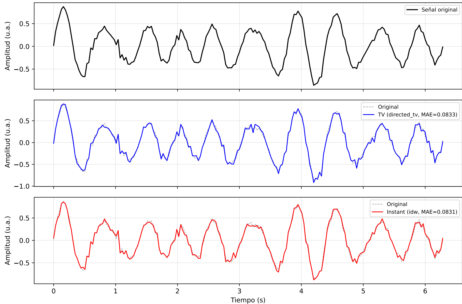
it17_synthetic_broad_all_graphs — Señal EEG: Original vs Reconstrucción
